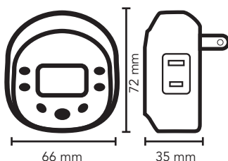
Type B plug Nema 5, 3 pole USA
